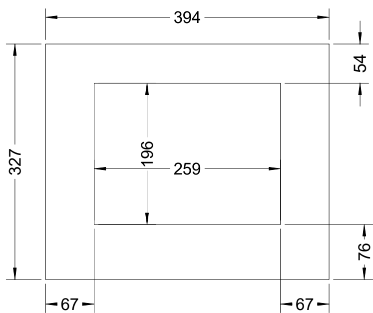
Door Frame
